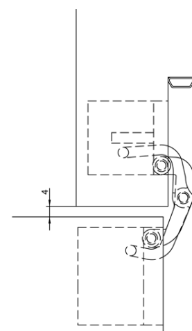
блочная дверная коробка 180°
