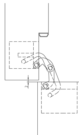
блочная дверная коробка 90°
