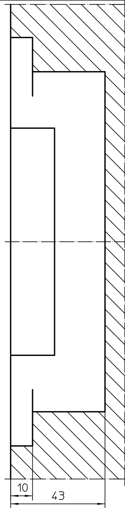
Fräsbild Flügel
