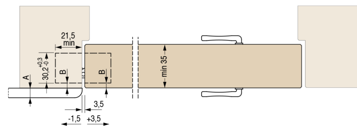
Разрез двери
