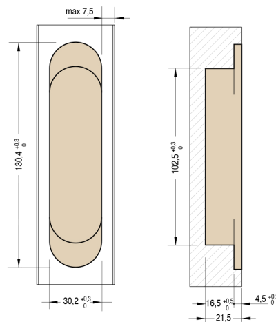
Размеры паза
